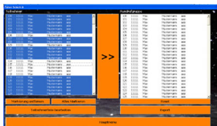
Screenshot BSR-Anwenderoberfläche
